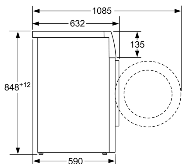
尺寸 (毫米)
