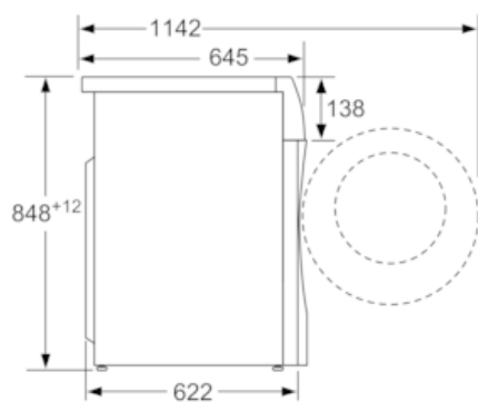
尺寸(毫米)
