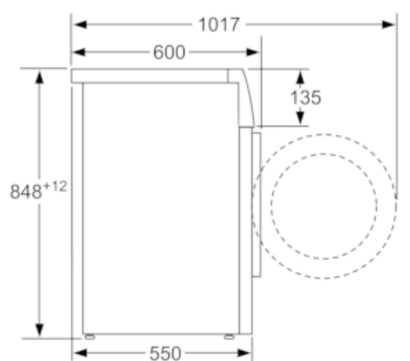
尺寸(毫米)
