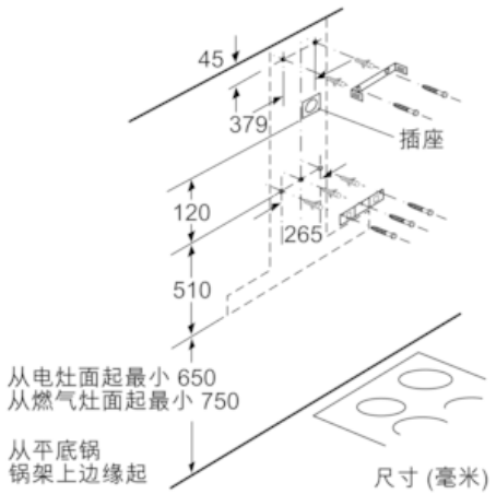
尺寸 (毫米)
