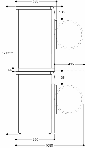
Ölçüler mm cinsindendir
