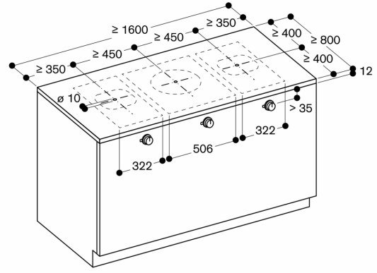
Ölçüler mm cinsindendir
