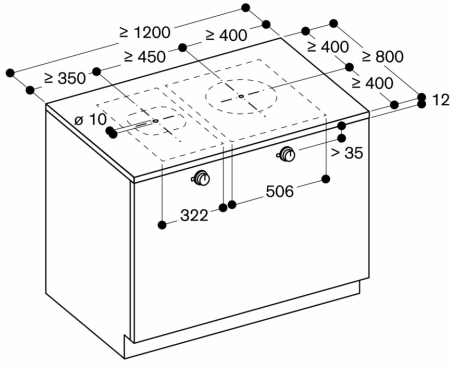
Ölçüler mm cinsindendir
