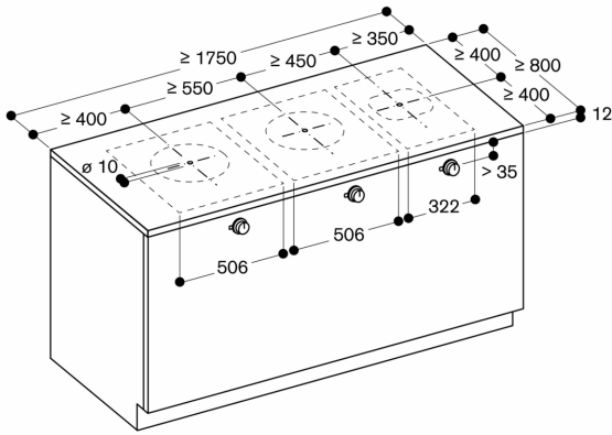
Ölçüler mm cinsindendir
