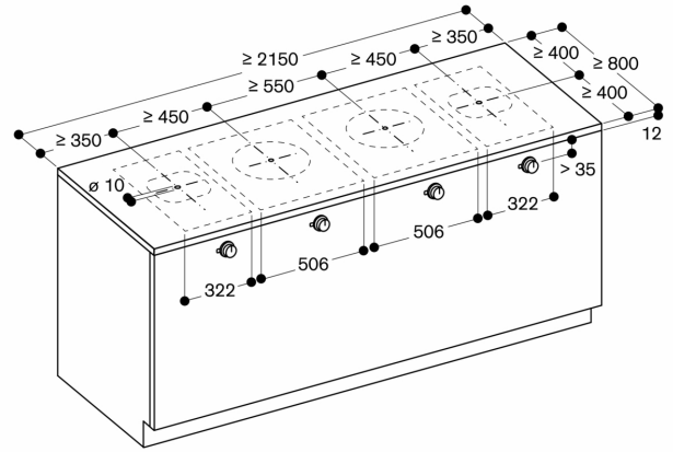
Ölçüler mm cinsindendir
