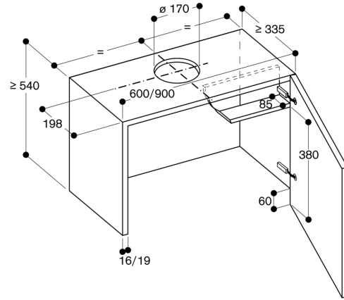
Alçaltma çerçevesi AF 210 için üst kabin
