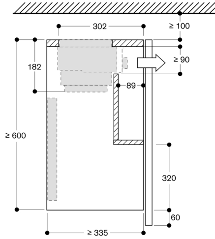
AA 211 812 ve AA 210 492/460 alçaltma çerçevesi AF210 için üst kabin çapraz kesiti
