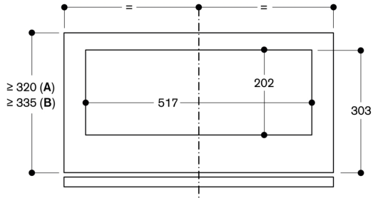
AA 211 812'li tezgah üstü dolabının yukarıdan görünümü
