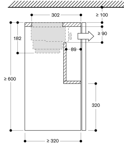
AA 211 812 ile AF210 için üst kabin çapraz kesiti
