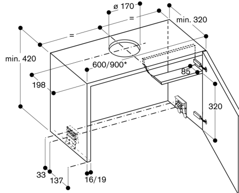
AF 210 için tezgah üstü dolabı
