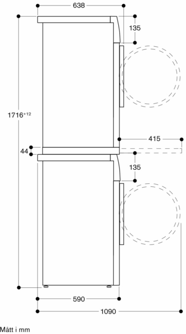
Sidovy av WT 260 ovanpå WM 260 med tillbehöret pelarmonteringsats
