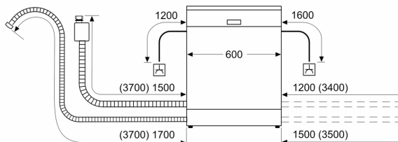
⌘ Eluttag ( ) mått med förlängningssats
