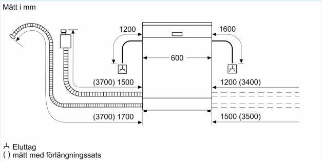
Måttskisser
