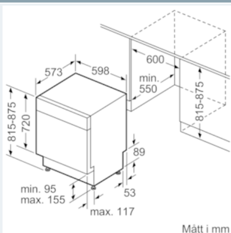
Måttskisser
