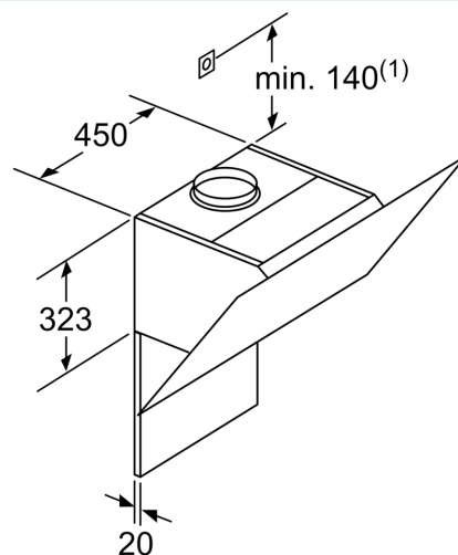
Mått i mm
