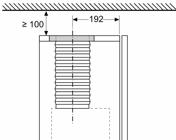
Mått i mm Installation av integrerad designkåpa med cirkulationssats (tillbehör)
