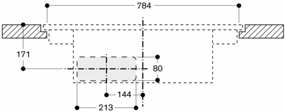
Frontvy – stomurtag för kanallös luftcirkulation; planmontering (CA 082 010)
