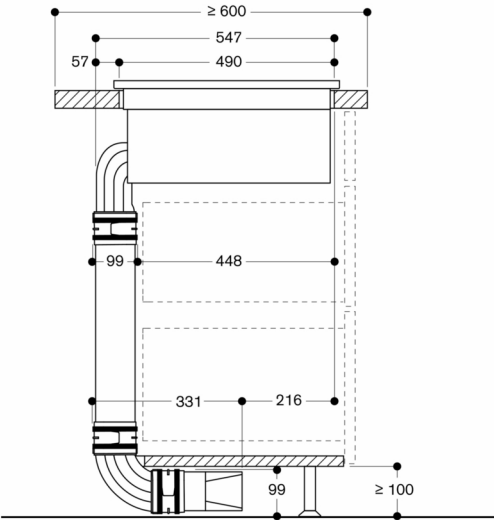
Sidovy med luftcirkulationskanalsats, 600 mm bänkskivdjup; utanpåliggande montering
