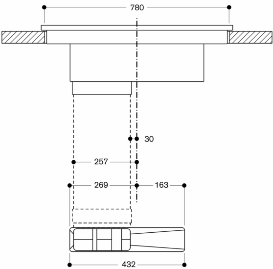
Frontvy av CV 282 med luftcirkulationskanalsats
