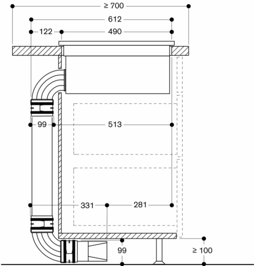
Sidovy med luftcirkulationskanalsats, 700 mm bänkskivdjup; utanpåliggande montering
