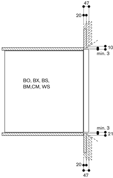
Ventilationsarea vid övre/undre luckkant
