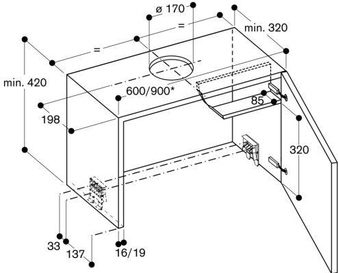
Överskåp till AF 210
