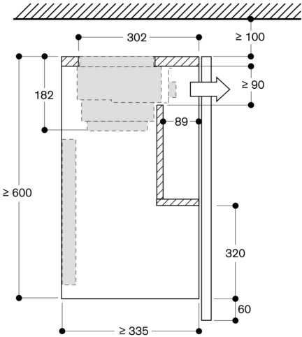
Tvärsnitt överskåp till AF210 med AA 211 812 och AA 210 492/460 nedsänkingsram
