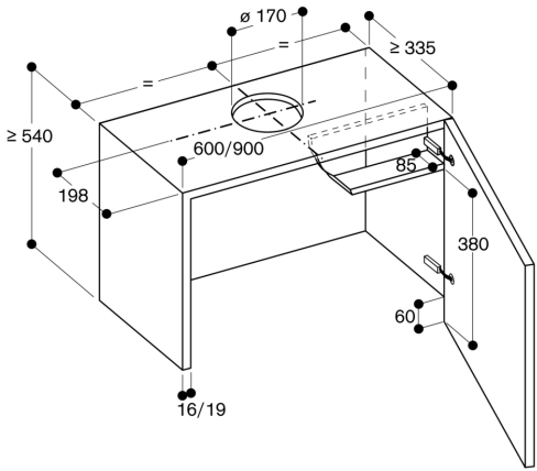
Överskåp till AF 210 med nedsänkingsram
