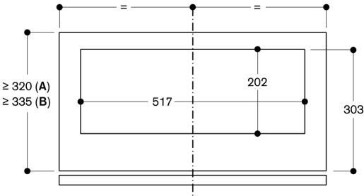
Vy ovanifrån, överskåp med AA 211 812
