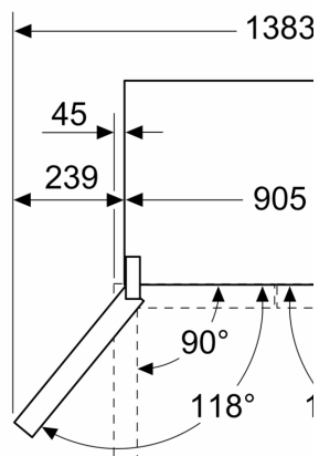
Dimenzije v mm
