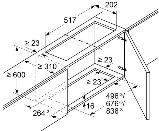
Dimenzije v mm Montaža popolnoma vgradne nape s kompletom za recirkulacijo zraka
