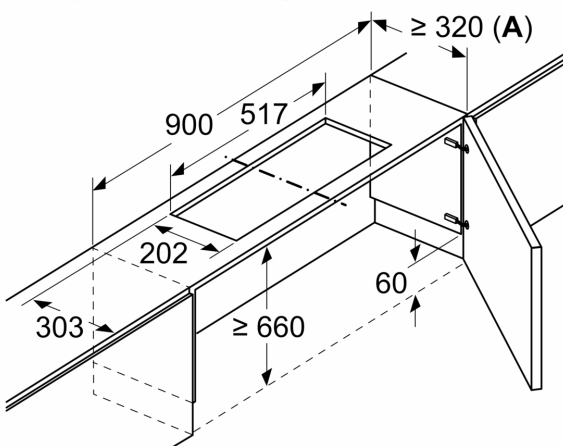
Dimenzije v mm Montaža vgradne izvlečne nape s kompletom za recirkulacijo zraka in okvirjem za skrito vgradnjo
