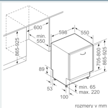
Rozmerové výkresy
