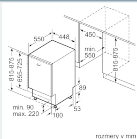
Rozmerové výkresy
