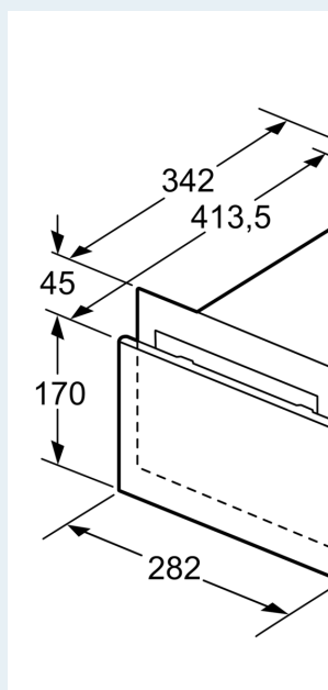
Rozmerové výkresy
