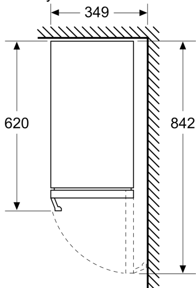
rozmery v mm
