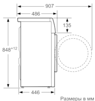
Размерные чертежи
