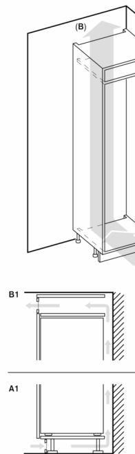
A: Abertura para admissão de ar \geq 200 cm 2 B: Abertura para saída de ar \geq 200 cm 2
