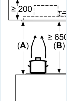
Medidas em mm Circulação de ar
