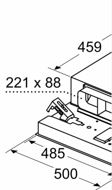
Medidas em mm
