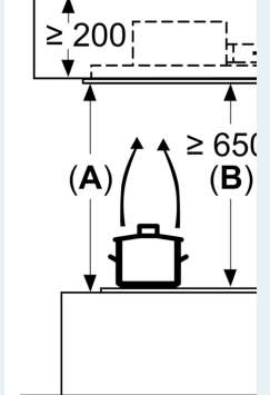
Medidas em mm Circulação de ar
