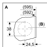
B: Otwór na zawias o głębokości min. 12 mm
