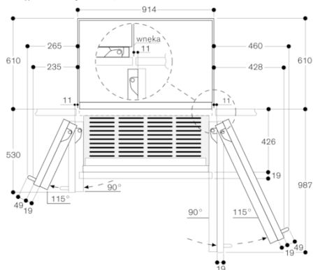
Odstęp od ściany RB 492/RY 492
