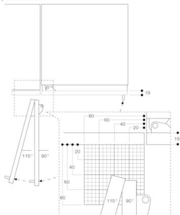
Kąt otwarcia drzwi
