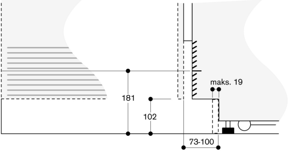
Detalj sokkel
