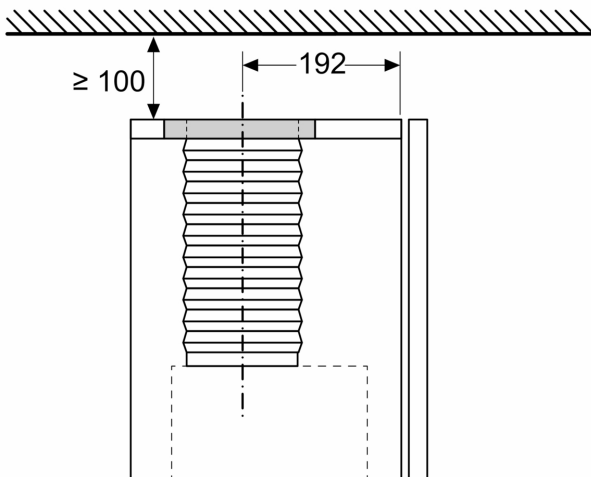
Mål i mm Montering av integrert ventilator med sirkulasjonssett (tilbehør)
