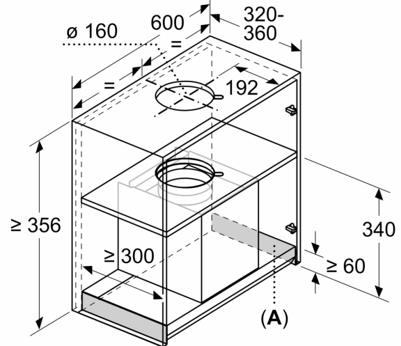
Mål i mm Eksempel på montering
