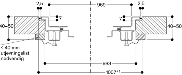
Lengdesnitt
