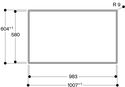
Sett ovenfra
