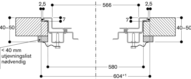
Tverrsnitt
