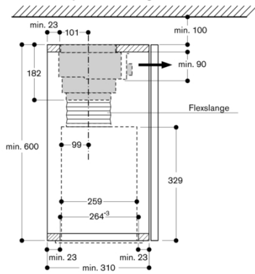
Tverrsnitt overskap med AC 200 og AA 211 812
