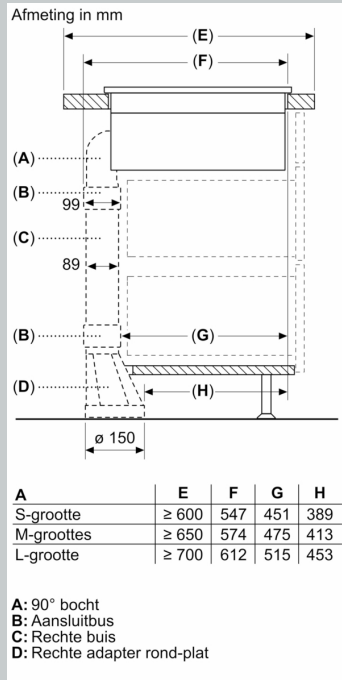
Afmeting in mm
