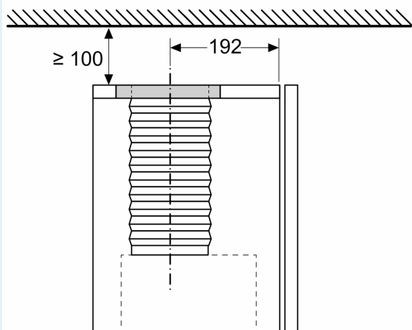
Afmeting in mm Installatie van geïntegreerde design afzuigkap met recirculatieset (accessoire)
