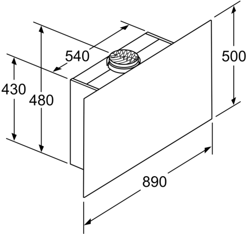
Apparaat in circulatiemodus zonder kanaal Circulatieset nodig Afmeting in mm
