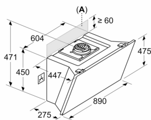
Afmeting in mm Apparaat in luchtcirculatiemodus zonder kanaal
