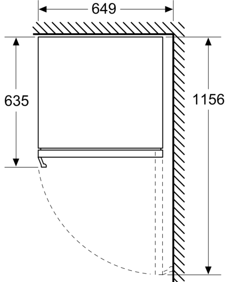
Afmeting in mm
