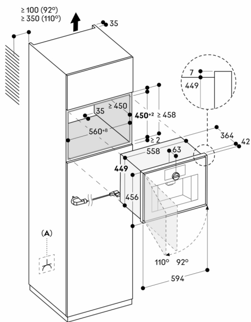
A: Toegankelijke elektrische aansluiting Afmeting in mm
