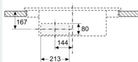
Afmeting in mm Vooranzicht - Meubeluitsparing voor circulatielucht zonder kanaal
