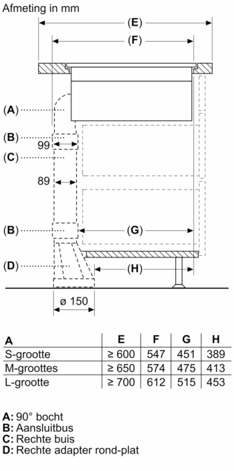
Afmeting in mm Vooraanzicht
