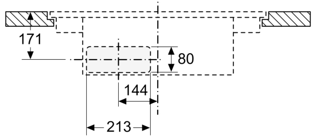
Afmeting in mm Vooraanzicht – unit uitsparing voor recirculatie zonder kanaal
