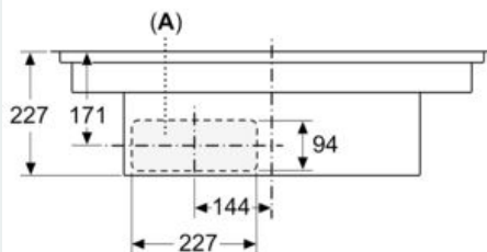
Afmeting in mm Voorraanzicht
