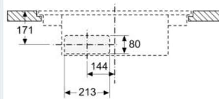
Voorraanzicht – unit uitsparing voor recirculatie zonder kanaal
