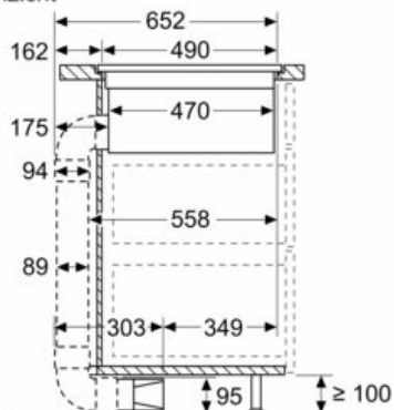
Afmeting in mm Zijaanzicht
