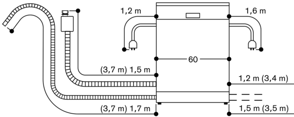
Aansluitmaten voor een 60 cm brede vaatwasser
