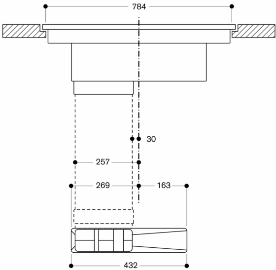
Frontaanzicht van CV 482 met kanaal-luchtrecirculatie
