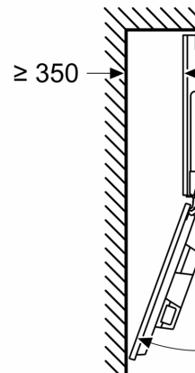
Afmeting in mm Installatie in link
