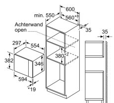
Afmeting in mm
