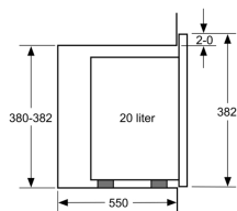
Afmeting in mm
