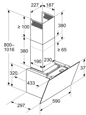
Afmeting in mm Apparaat in luchtcirculatiemodus
