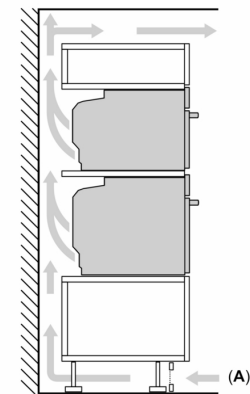
Inbouw van twee apparaten boven elkaar Luchtverversing
