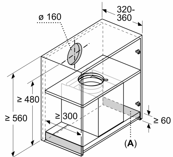
Izmēri mm
