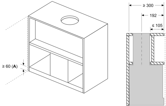
Izmēri mm Instalācijas piemērs ar garšvielu plauktu
