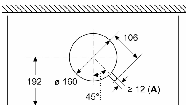
Izmēri mm Virsskats
