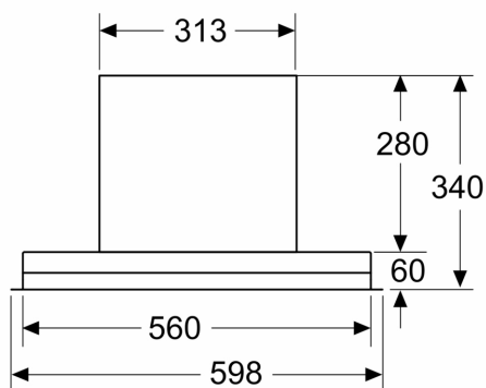
Izmēri mm Skats no priekšas
