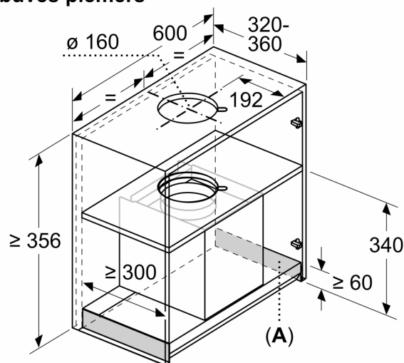
Izmēri mm Iebūves piemērs
