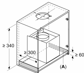
Izmēri mm Uzstādīšanas prasības nomaināmas darbībām
