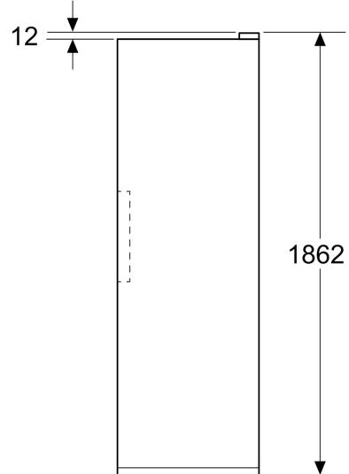
Matmenys, mm
